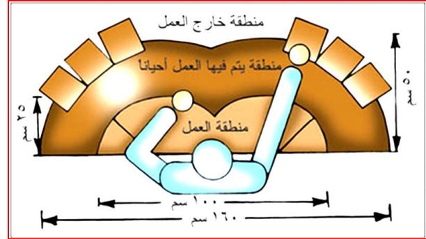
شكل رقم (2) مدى حدود حركة اليد للعامل على منضدة العمل
